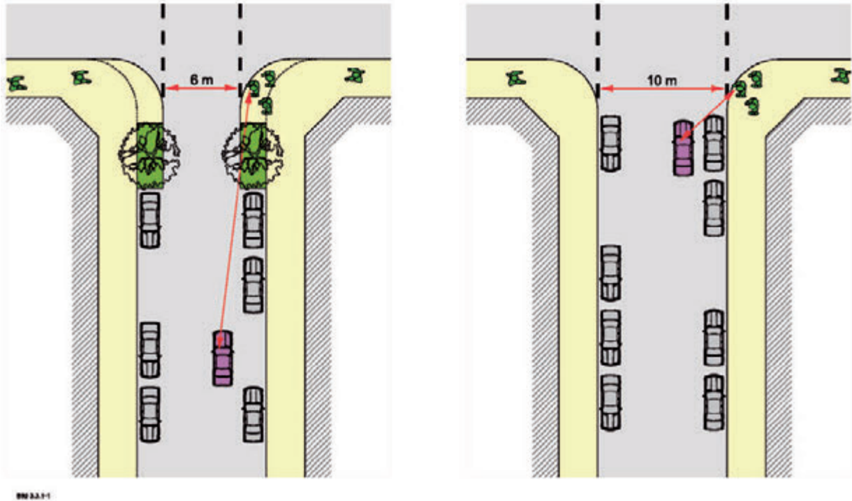
Abb. 12: links: mit Gehwegnase - große Sichtweite/kurze Querungslänge, rechts: ohne Gehwegnase - kurze Sichtweite/lange Querungslänge, Quelle: H. Stadt (2012).
